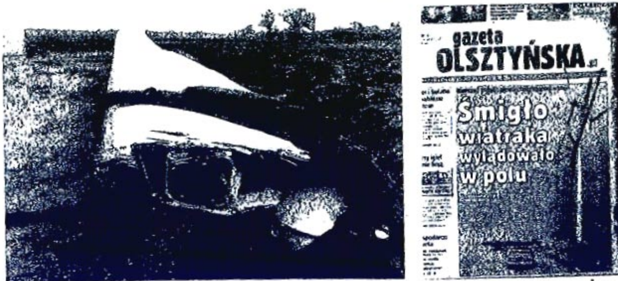
Rys. 9. Łopata na farmie w Korszach, z której urwała się 5.5 metrowa końcówka.
