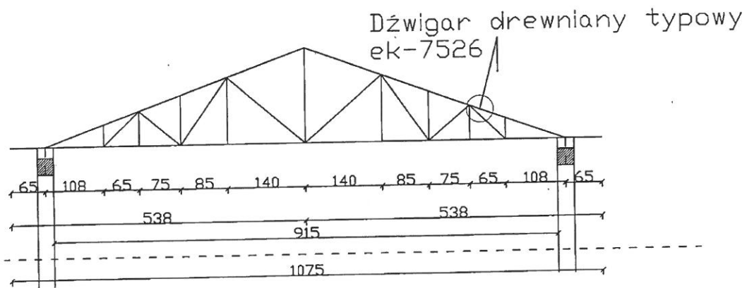
PRZEKRÓJ A-A OSP PODGÓRZE
